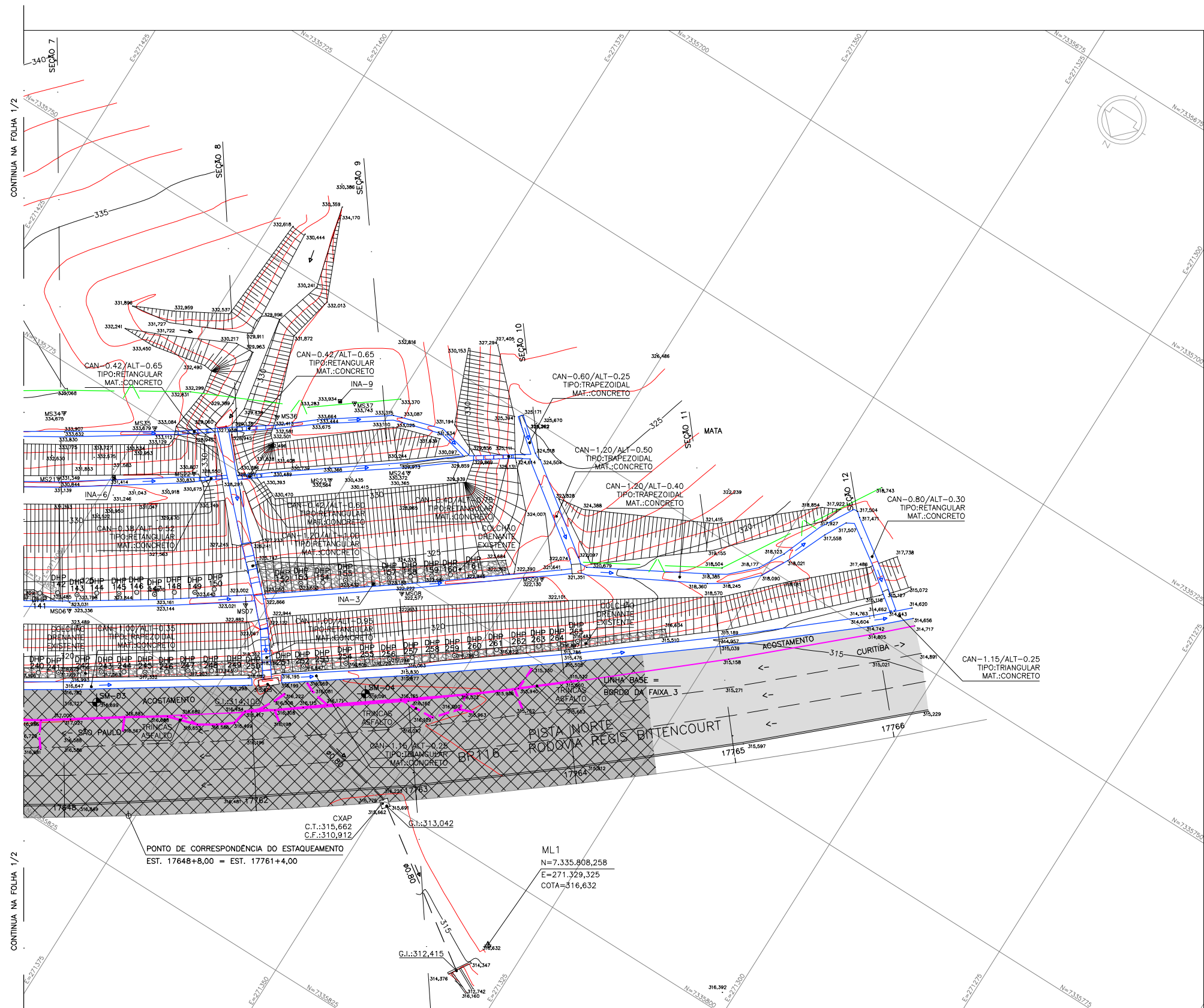
PLANTA DE DISTRIBUIÇÃO DE PAVIMENTO – FOLHA 2/2 ESCALA 1:250
